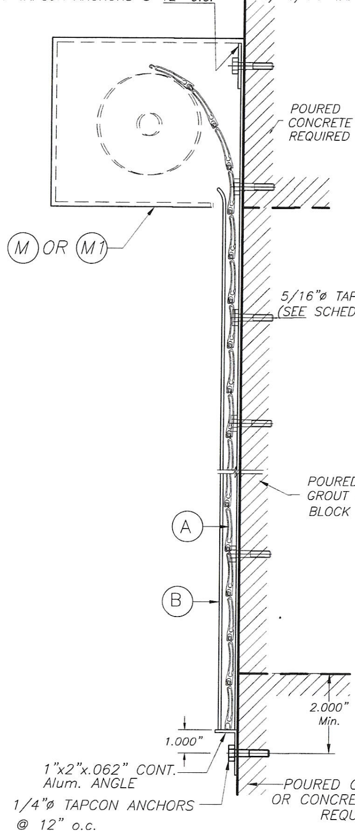
SECTION P-P (1) N. T. S.
